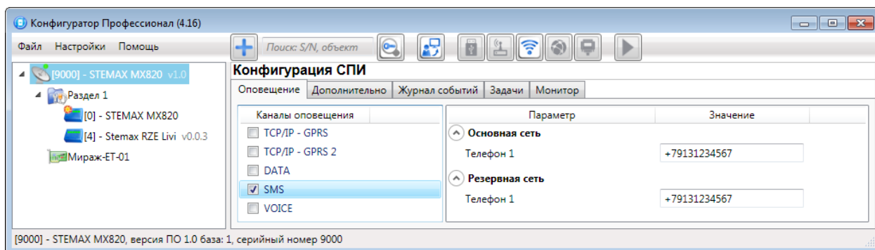
Рис. 5.9. Параметры канала SMS
