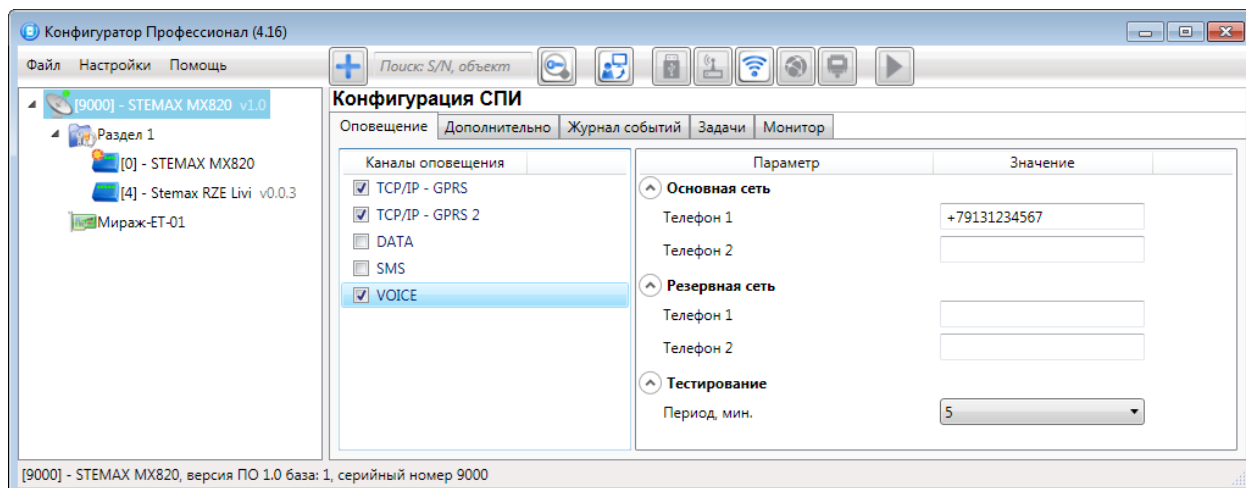
Рис. 5.10. Параметры канала VOICE
