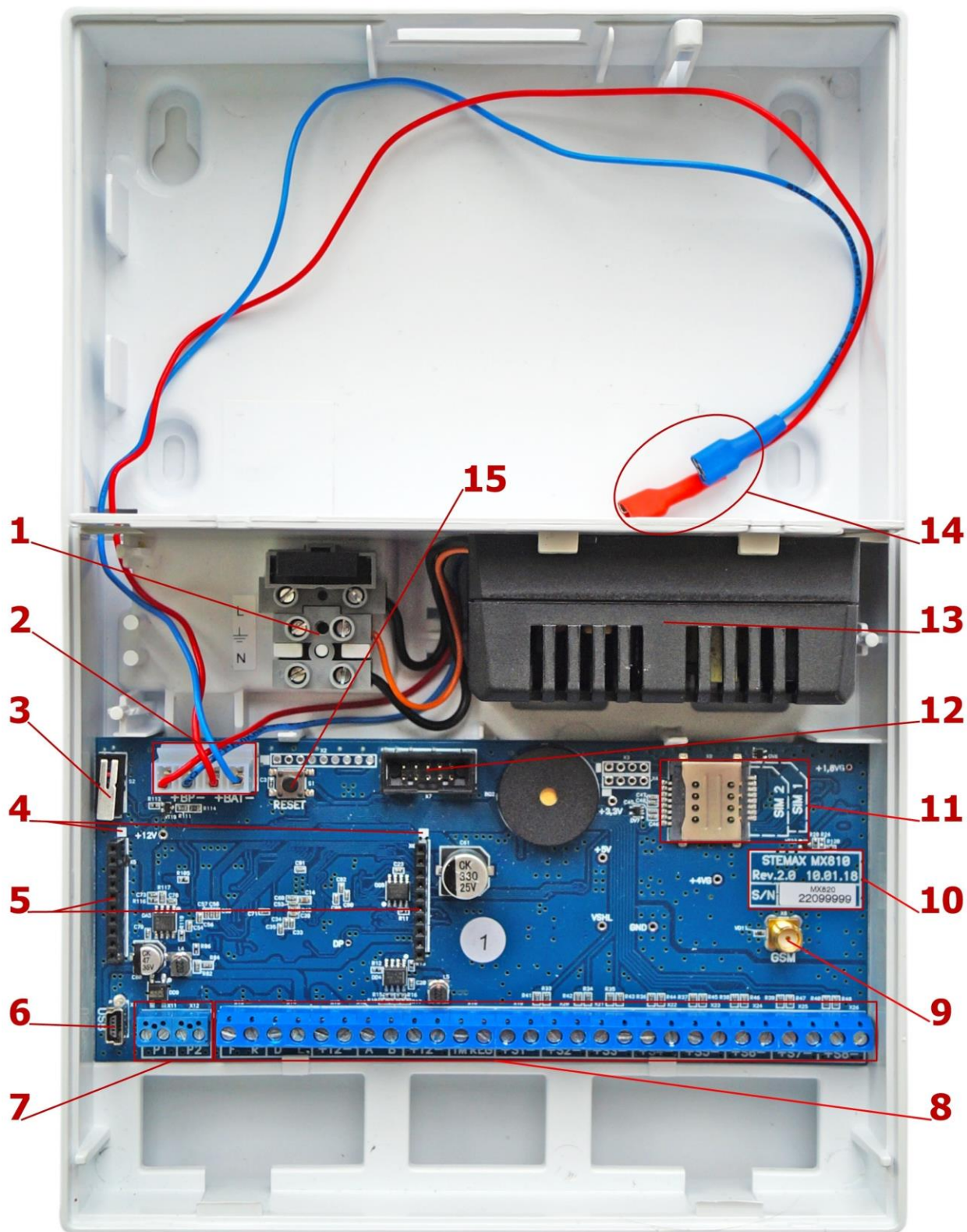
Рис. 10.1. Вид контроллера со снятой крышкой
