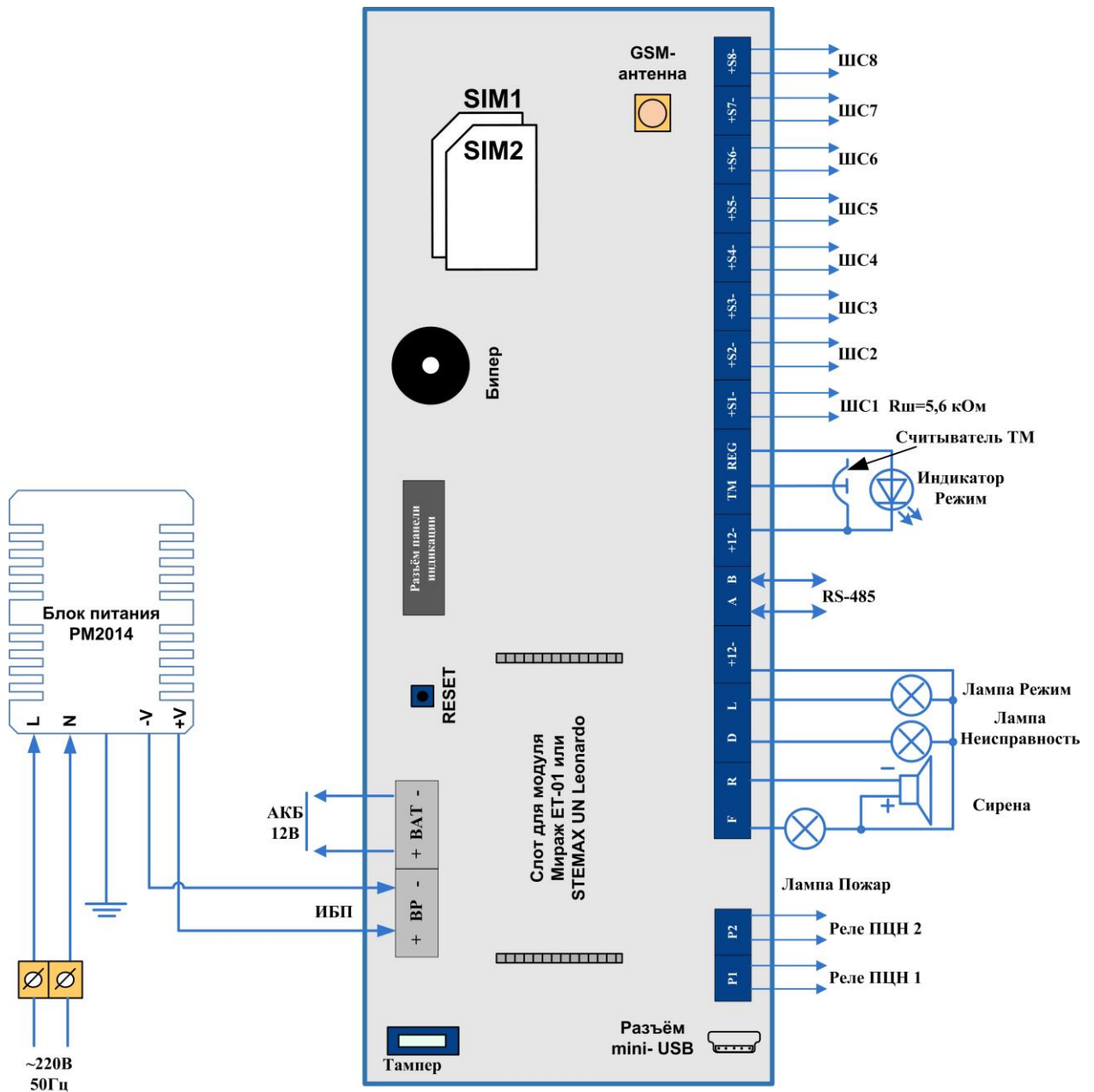
Рис. 10.2. Схема внешних подключений контроллера
