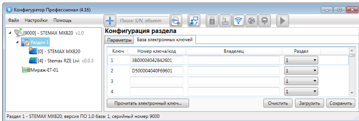
Рис. 5.21. Вкладка База электронных ключей
