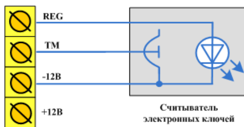
Рис. 7.1. Схема подключения считывателя Touch Memory
