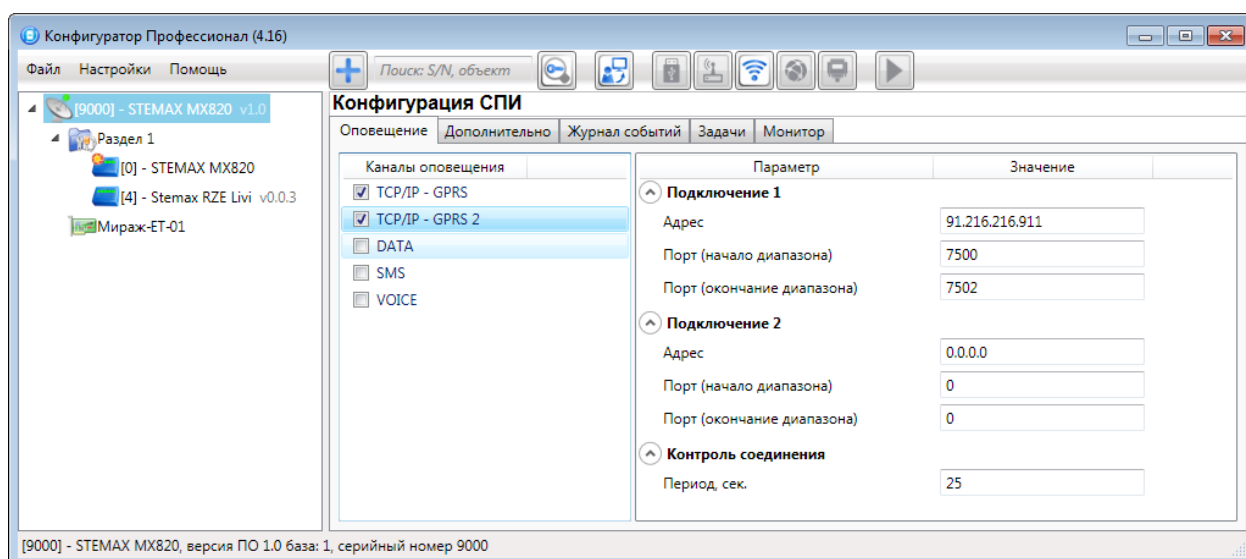
Рис. 5.7. Параметры канала TCP/IP GPRS 2
