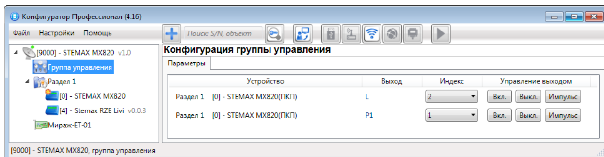
Рис. 5.31. Параметры и элементы дистанционного управления
